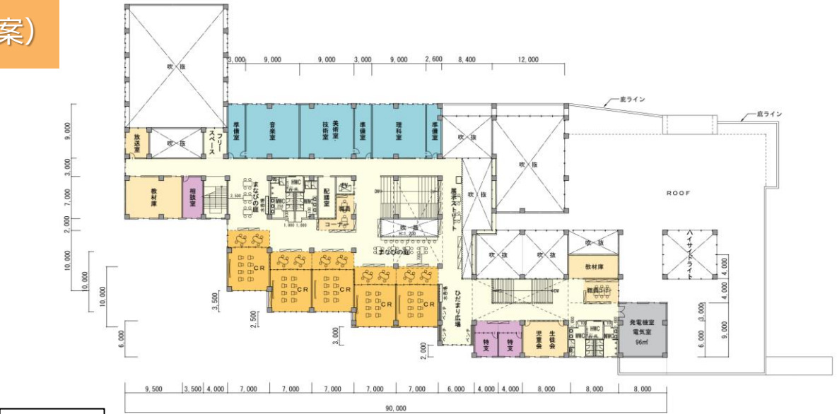
2階平面図
